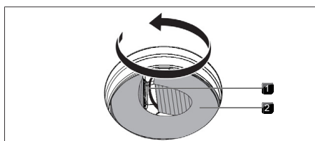
Fig. 9.5 Rodar o filtro de carvão ativado da carcaça do filtro
