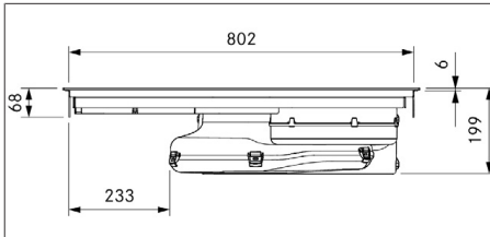
Fig. 3.5 PUXU2/R dimensões do aparelho vista frontal
