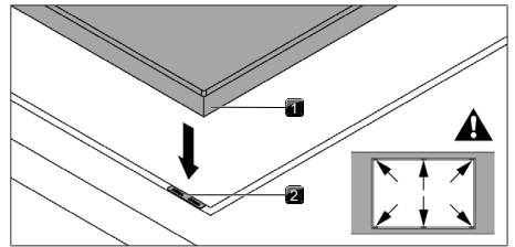
Fig. 11.21 Posicionamento e placas de compensação de altura
