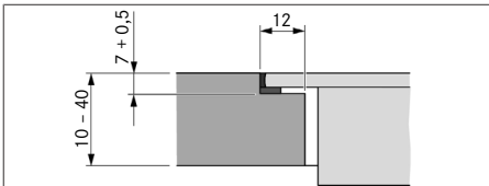
Fig. 11.6 Medida de recesso para montagem à face
