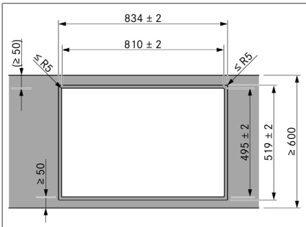
Fig. 11.5 Medidas de recorte para montagem à face
