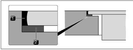
Fig. 11.18 Cinta vedante na montagem à face
