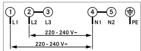
Fig. 11.29 Esquema de ligações bifásico
