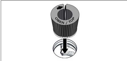
Fig. 9.8 Inserir o filtro de carvão ativado na abertura do exaustor
