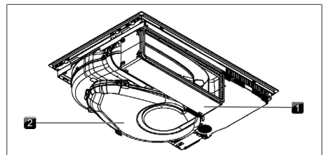
Fig. 4.3 Vista traseira da versão com sistema de circulação de ar
