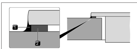
Fig. 11.17 Cinta vedante para montagem por sobreposição
