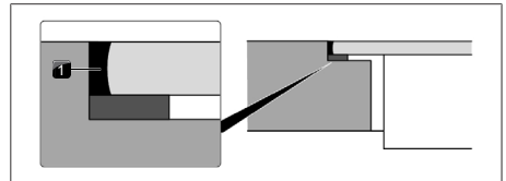
Fig. 11.36 Massa vedante de silicone na montagem à face
