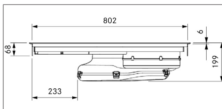
Fig. 3.2 PUXA2/R dimensões do aparelho vista frontal
