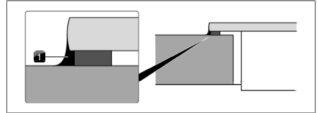
Fig. 11.35 Massa vedante de silicone na montagem por sobreposição
