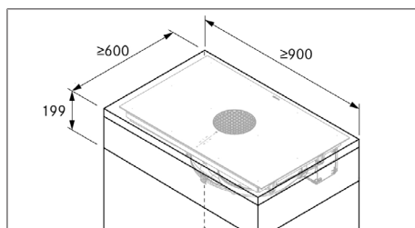
obr. 10.4 Minimální rozměry nábytku – X Pure
