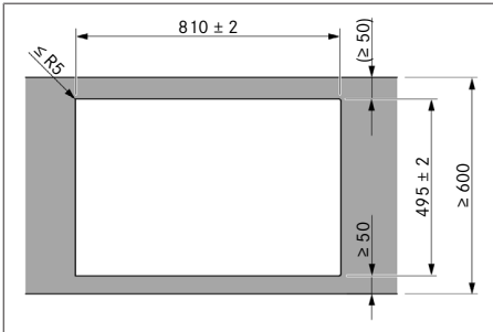
obr. 10.7 Rozměry výřezu pro montáž na povrch
