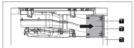
obr. 10.25 Přípojka k zadní stěně
