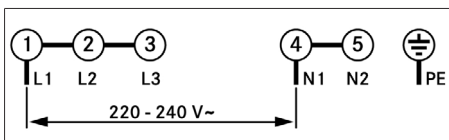
obr. 10.28 Schéma zapojení 1fázové přípojky
