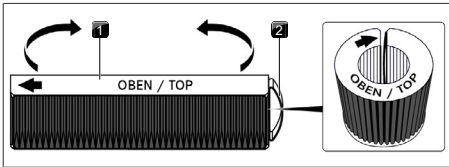
obr. 8.7 Filtr s aktivním uhlím
