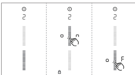
obr. 7.3 Položka nabídky 2: Dětská pojistka
