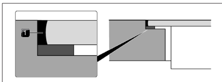
obr. 10.36 Silikonová těsnicí hmota při plošně zarovnané montáži
