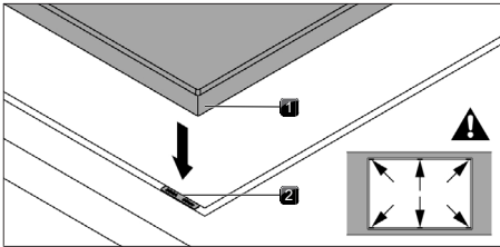
obr. 10.21 Pozice podložek k nastavení výšky
