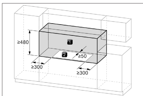
obr. 10.3 Požadovaný volný prostor
