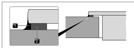
obr. 10.17 Těsnicí páska při montáži na povrch
