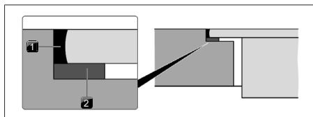
obr. 10.18 Těsnicí páska při plošně zarovnané montáži
