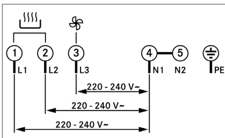
obr. 10.27 Schéma zapojení 3fázové přípojky
