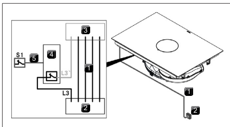
obr. 10.26 Schéma zapojení s externím spínacím kontaktem
