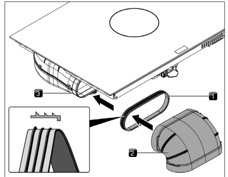
obr. 10.24 Připojení systému odtahových potrubí
