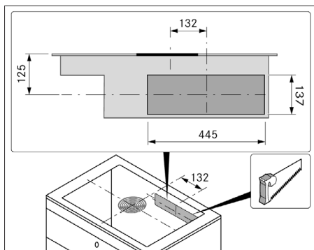
obr. 10.11 Výřez v zadní stěně
