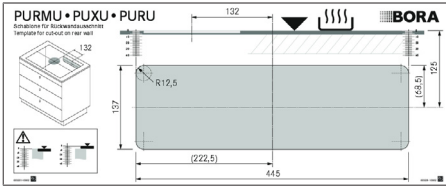
obr. 10.12 Šablona pro výřez zadní stěny
