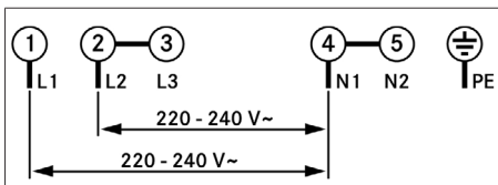
obr. 10.29 Schéma zapojení 2fázové přípojky
