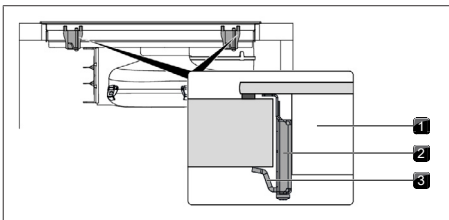
obr. 10.23 Upevnění varné desky do středu
