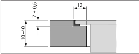
obr. 10.6 Rozměr drážky pro plošně zarovnanou montáž
