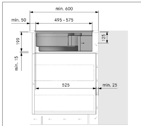
obr. 10.16 Rozměry montáže u varianty montáže B, hloubka pracovní desky 600 mm
