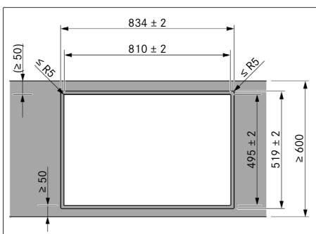
obr. 10.5 Rozměry výřezu pro plošně zarovnanou montáž
