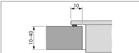
obr. 10.8 Rozměry podkladu pro montáž na povrch
