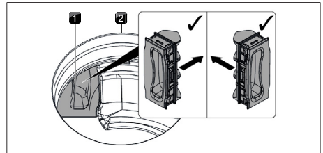
obr. 8.10 Nasazení výměnné klapky filtru
