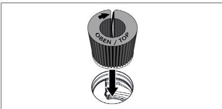
obr. 8.8 Nasazení filtru s aktivním uhlím do otvoru odsavače
