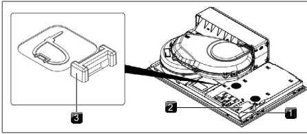
obr. 10.30 Elektrické přípojky varné desky
