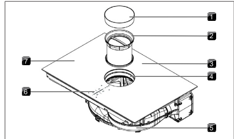
obr. 4.1 Uspořádání
