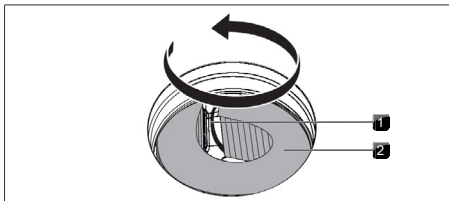
obr. 8.5 Vyšroubování filtru s aktivním uhlím ze skříně filtru
