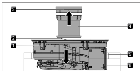
obr. 10.20 Upevnění varné desky do středu
