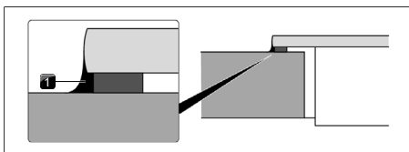
obr. 10.35 Silikonová těsnicí hmota při montáži na povrch
