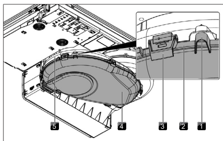
obr. 8.3 Skříň ventilace
