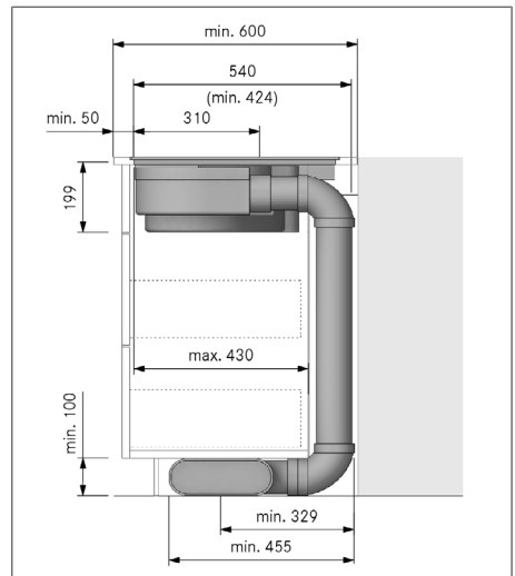
obr. 10.9 Rozměry montáže při odtahu ven, hloubka pracovní desky 600 mm
