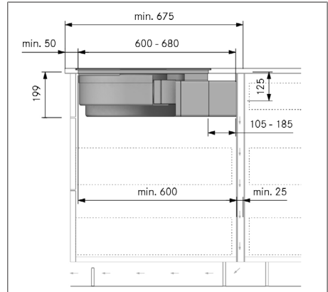
obr. 10.14 Rozměry montáže u varianty montáže A, hloubka pracovní desky od 675 mm
