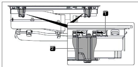
obr. 10.19 Umístění montážních svorek
