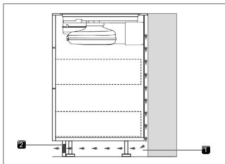
obr. 10.10 Otvor na zpětné proudění vzduchu v oblasti soklu
