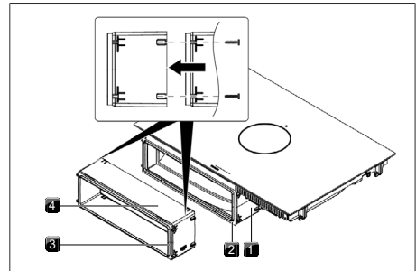
obr. 10.15 Nastavení teleskopického výsuvu
