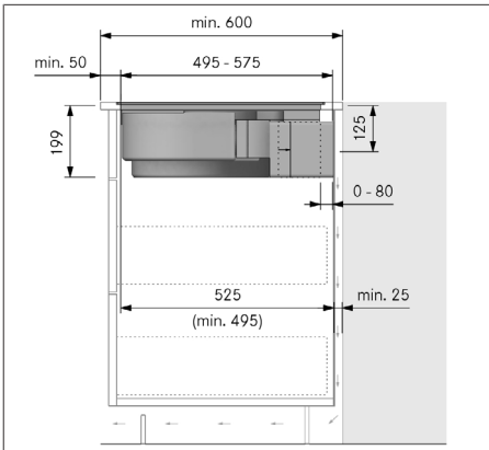
obr. 10.13 Rozměry montáže u recirkulujícího vzduchu, varianta montáže A
