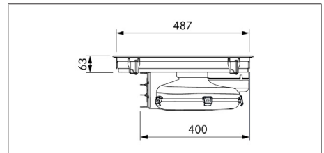
Fig. 3.3 Dimensions PUXA2/R - Vue latérale
