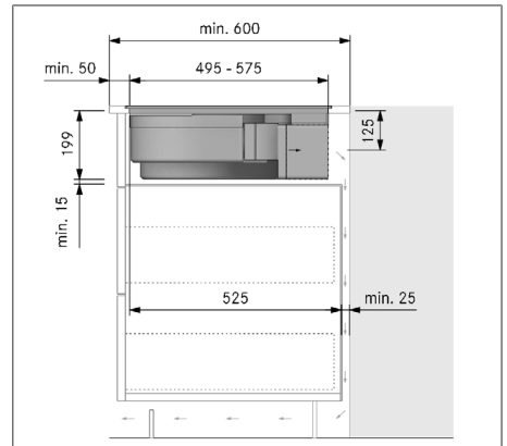
Fig. 11.16 Cotes de montage pour le recyclage d'air, variante B, profondeur du plan de travail 600 mm
