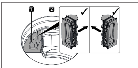
Fig. 9.10 Pose du clapet de changement de filtre
