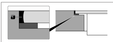
Fig. 11.36 Joint en silicone en montage affleurant
