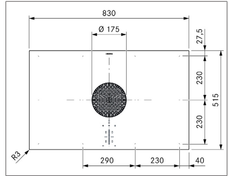
Fig. 3.1 Dimensions PUXA2/R - Vue de dessus
