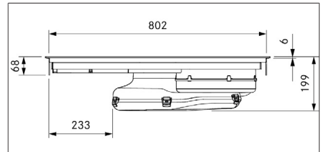
Fig. 3.2 Dimensions PUXA2/R - Vue de devant
