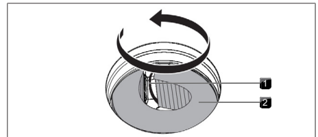
Fig. 9.5 Rotation du filtre à charbon actif dans son boîtier
