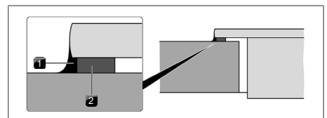
Fig. 11.17 Ruban d'étanchéité pour montage en saillie
