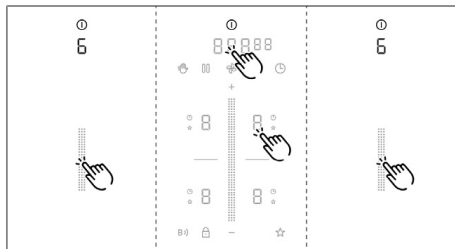
Fig. 8.7 Option de menu 6 : test des LED
