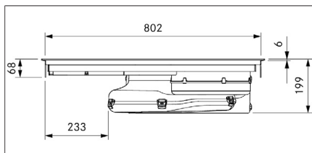
Fig. 3.5 Dimensions PUXU2/R - Vue de devant
