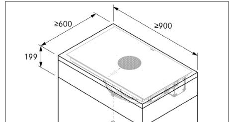
Fig. 11.4 Dimensions minimales du meuble pour X Pure
