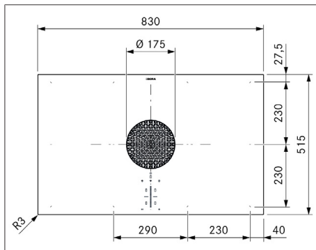
Fig. 3.4 Dimensions PUXU2/R - Vue de dessus
