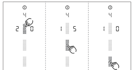
Fig. 8.5 Option de menu 4 : sélection de la durée de la temporisation automatique
