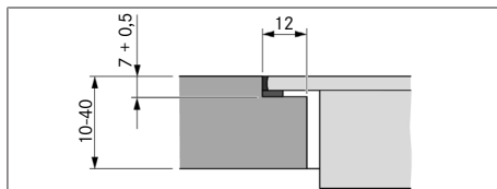
Fig. 11.6 Dimensioni dell'incassatura per montaggio a filo piano
