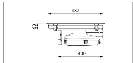
Fig. 3.3 PUXA2/R dimensioni apparecchio vista laterale
