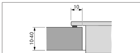
Fig. 11.8 Misura d'appoggio per montaggio in battuta
