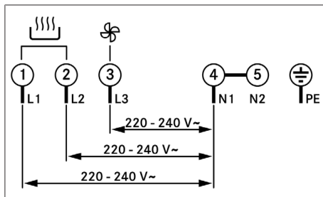
Fig. 11.27 Schema di collegamento collegamento trifase
