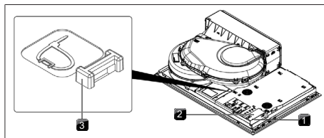
Fig. 11.30 Collegamenti elettrici del piano cottura
