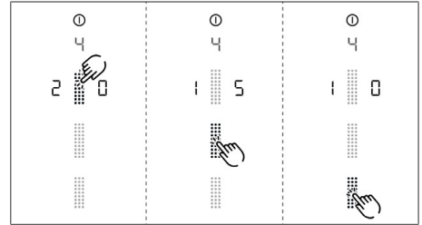
Fig. 8.5 Voce di menu 4: Selezionare la durata della funzione di spegnimento automatico ritardato
