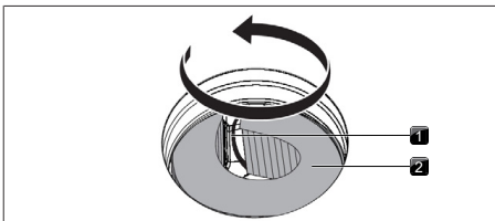
Fig. 9.5 Ruotare il filtro al carbone attivo dalla cassetta del filtro
