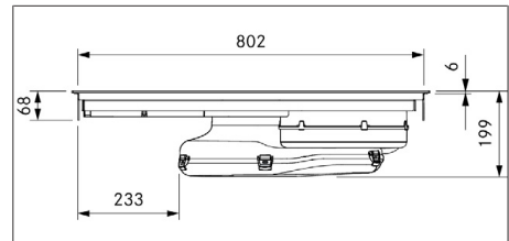
Fig. 3.2 PUXA2/R dimensioni apparecchio vista frontale
