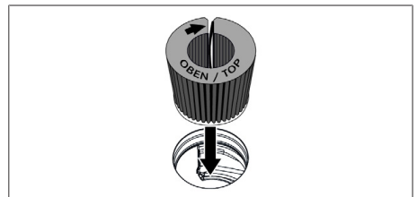
Fig. 9.8 Inserire il filtro al carbone attivo nell'apertura di aspirazione
