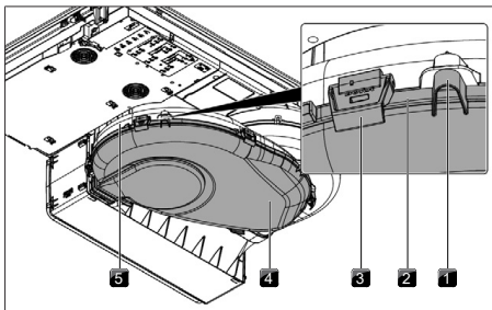
Fig. 9.3 Alloggiamento condotta aria
