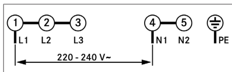
Fig. 11.28 Schema di collegamento collegamento monofase
