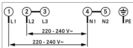
Fig. 11.29 Schema di collegamento collegamento bifase
