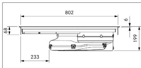
Fig. 3.5 PUXU2/R dimensioni apparecchio vista frontale
