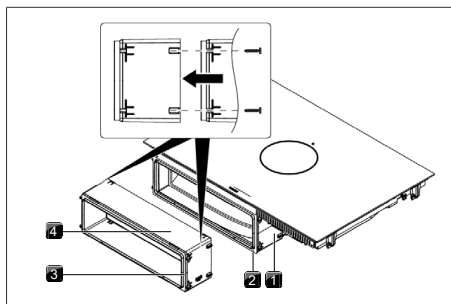
Fig. 11.15 Estensione della prolunga telescopica
