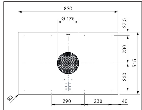
Fig. 3.1 PUXA2/R dimensioni apparecchio vista dall'alto
