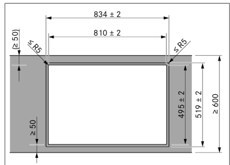
Fig. 11.5 Dimensioni intaglio per montaggio a filo
