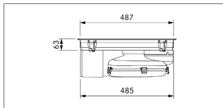
Fig. 3.6 PUXU2/R dimensioni apparecchio vista laterale
