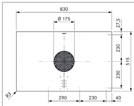
Fig. 3.4 PUXU2/R dimensioni apparecchio vista dall'alto
