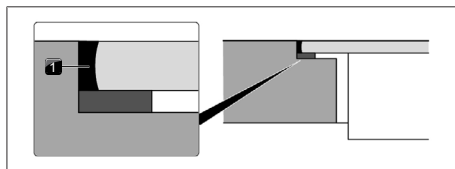
Abb. 10.36 Silikondichtmasse bei flächenbündiger Montage
