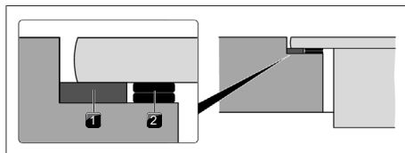
Abb. 10.22 Höhenausgleichsplatten
