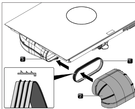
Abb. 10.24 Anschluss an Kanalsystem
