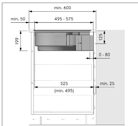
Abb. 10.13 Einbaumaße bei Umluft, Montagevariante A
