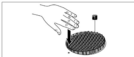
Abb. 8.1 Einströmdüse entnehmen
