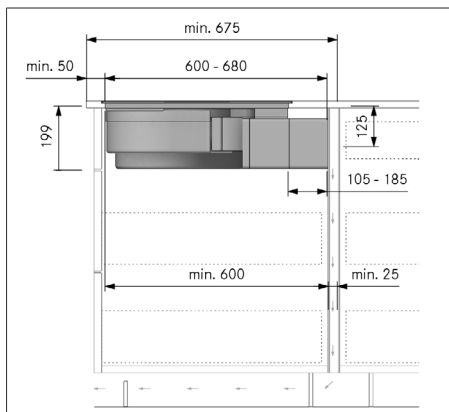
Abb. 10.14 Einbaumaße bei Umluft-Montagevariante A, Arbeitsplattentiefe ab 675 mm
