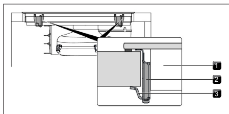
Abb. 10.23 Kochfeld mittig befestigen
