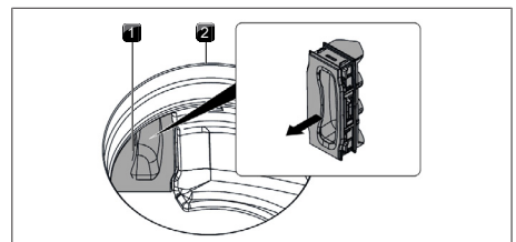
Abb. 8.4 Filterwechselklappe entfernen
