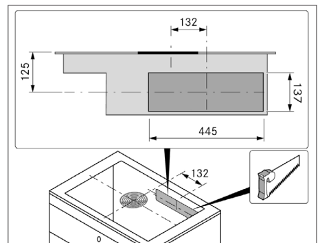
Abb. 10.11 Rückwand-Ausschnitt
