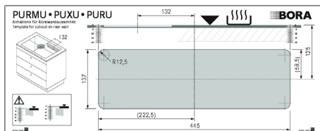
Abb. 10.12 Schablone für Rückwand-Ausschnitt
