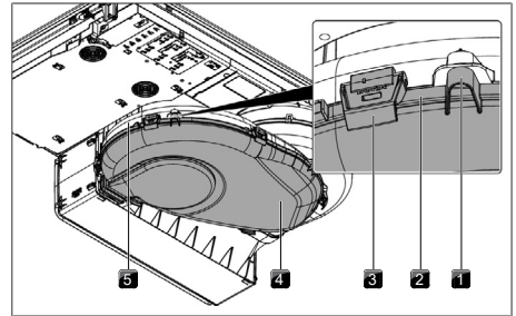
Abb. 8.3 Luftführungsgehäuse
