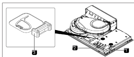
Abb. 10.30 Elektrische Anschlüsse des Kochfeldes
