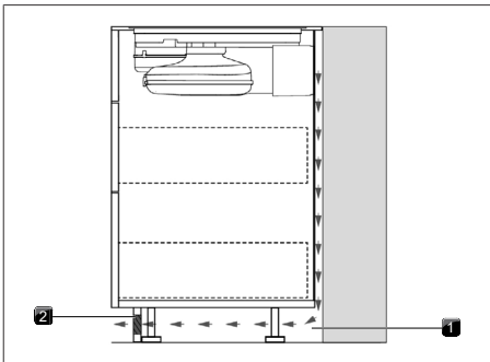
Abb. 10.10 Rückströmöffnung im Sockelbereich
