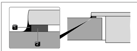
Abb. 10.17 Dichtungsband bei Aufsatzmontage
