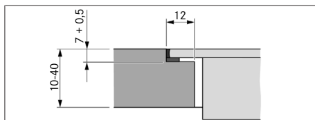
Abb. 10.6 Falzmaß für flächenbündige Montage
