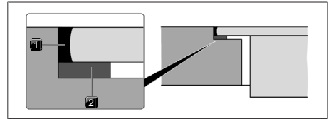
Abb. 10.18 Dichtungsband bei flächenbündiger Montage
