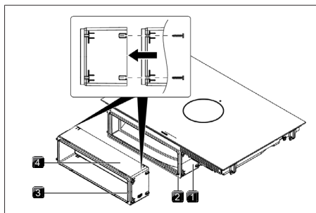
Abb. 10.15 Verlängerung des Teleskopauszuges
