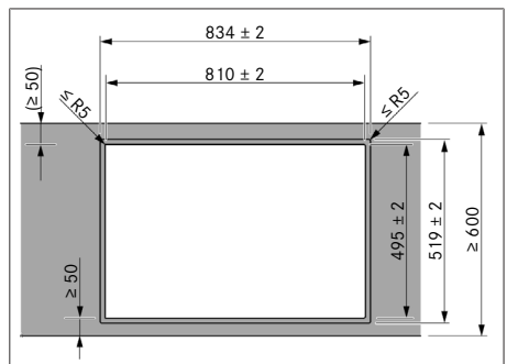
Abb. 10.5 Ausschnittsmaße für flächenbündige Montage
