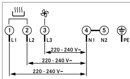
Abb. 10.27 Anschlusschema 3-Phasen-Anschluss
