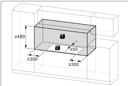
Abb. 10.3 Erforderlicher Freiraum
