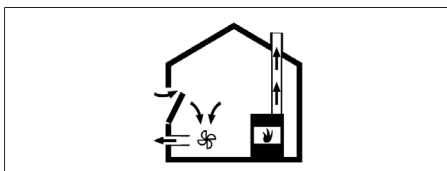
Abb. 10.2 Abluftmontage – korrekt
