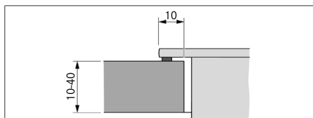
Abb. 10.8 Auflagemaß für Aufsatzmontage
