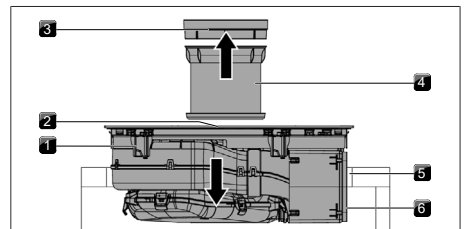
Abb. 10.20 Kochfeld mittig einsetzen
