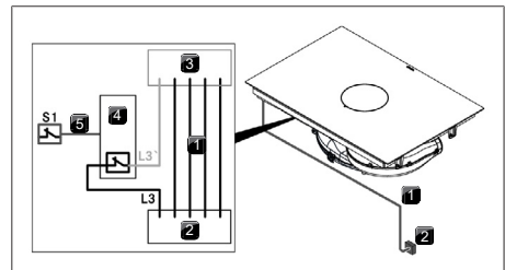
Abb. 10.26 Anschlussschema mit externem Schaltkontakt
