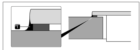
Abb. 10.35 Silikondichtmasse bei Aufsatzmontage
