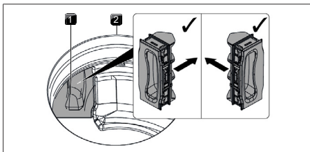
Abb. 8.10 Filterwechsellappe einsetzen
