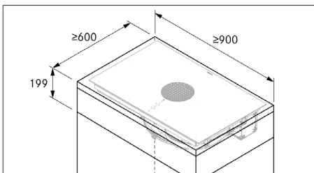
Abb. 10.4 Möbel-Mindestmaße X Pure
