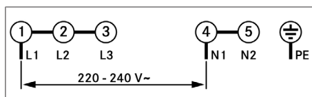
Abb. 10.28 Anschlusschema 1-Phasen-Anschluss
