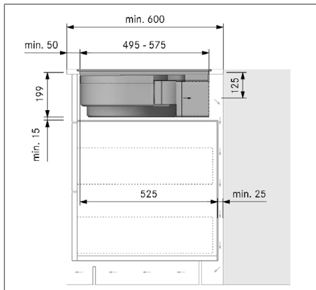
Abb. 10.16 Einbaumaße bei Umluft-Montagevariante B, Arbeitsplattentiefe 600 mm
