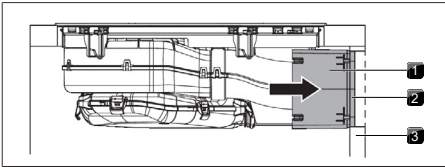
Abb. 10.25 Rückwandanschluss
