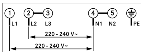
Abb. 10.29 Anschlusschema 2-Phasen-Anschluss
