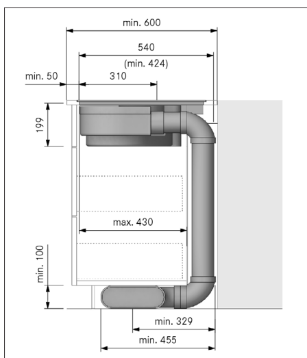
Abb. 10.9 Einbaumaße Abluft, Arbeitsplattentiefe 600 mm
