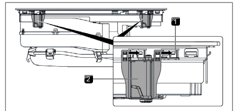
Abb. 10.19 Montageklammern anbringen
