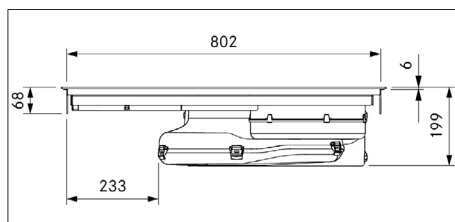
Abb. 3.5 PUXU2/R Gerätemaße Vorderansicht
