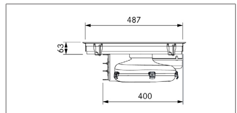
Abb. 3.3 PUXA2/R Gerätemaße Seitenansicht
