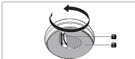
Abb. 8.5 Aktivkohlefilter aus dem Filtergehäuse drehen
