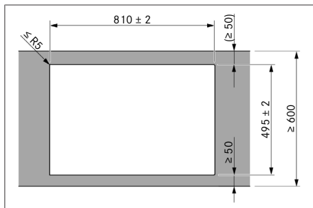
Abb. 10.7 Ausschnittsmaße für Aufsatzmontage
