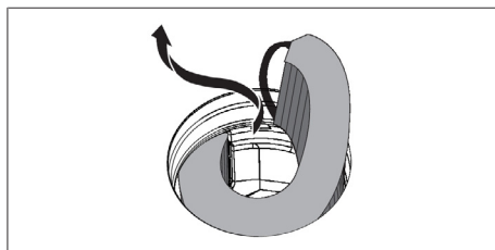
Abb. 8.6 Aktivkohlefilter aus der Einströmöffnung entnehmen
