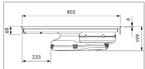
Abb. 3.2 PUXA2/R Gerätemaße Vorderansicht
