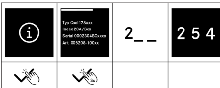
Abb. 7.12 Händlermenü öffnen
