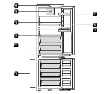
obr. 5.3 Uspořádání C178KG
