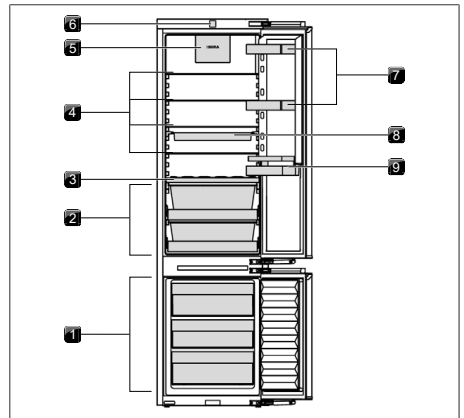
obr. 5.5 Uspořádání C194KG
