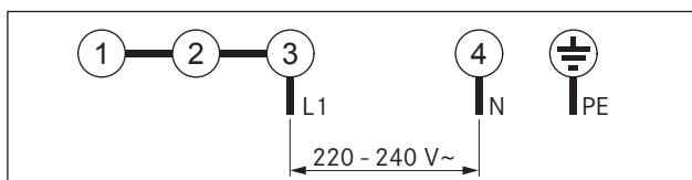
Fig. 6.38 Schéma de raccordement 1 phases de raccordement
