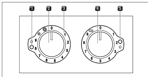
Sl. 4.4 Gumb za upravljanje PC3B
