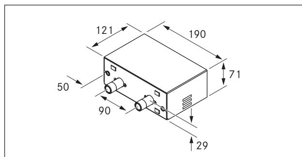
Sl. 3.3 Dimenzije električne omarice PC32/PC3B
