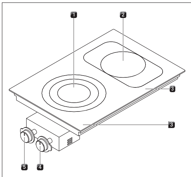
Sl. 4.2 Kuhalna plošča PC3B
