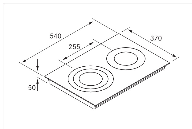
Sl. 3.1 Dimenzije naprave PC32
