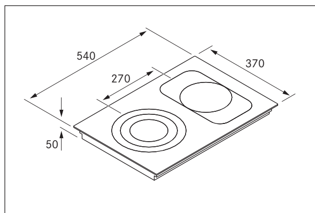
Sl. 3.2 Dimenzije naprave PC3B
