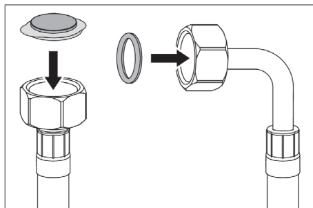
Fig. 9.13 Tubo di alimentazione dell'acqua con setaccio e guarnizione
