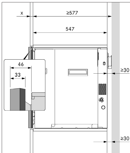
Fig. 9.4 Dimensioni di montaggio 1 distanziatori cornice
