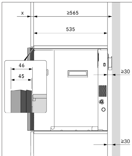
Fig. 9.5 Dimensioni di montaggio 2 distanziatori cornice
