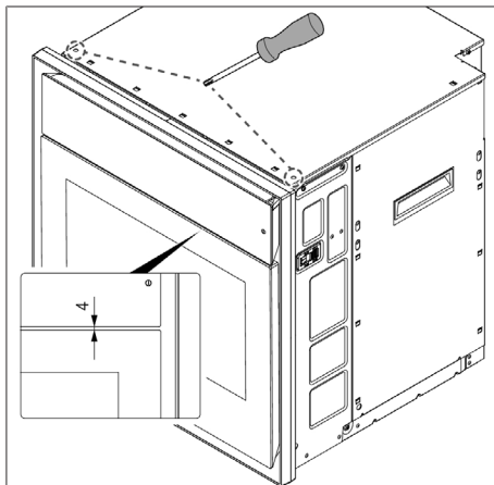
Fig. 9.15 Impostazione distanza unità di comando e porta
