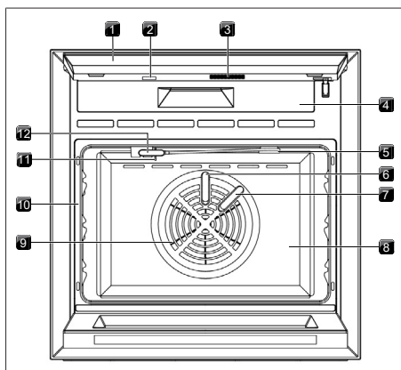
Fig. 4.1 Struttura parte 1
