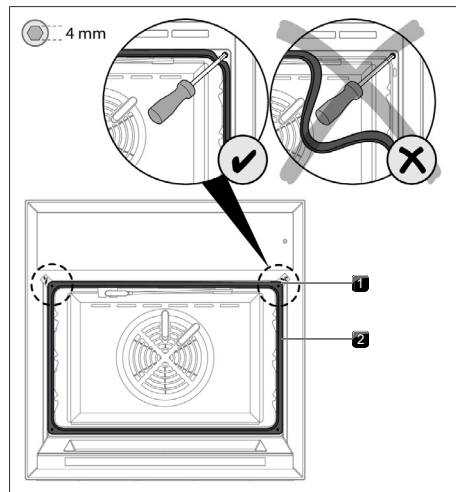
Fig. 9.16 Fissare l'apparecchio
