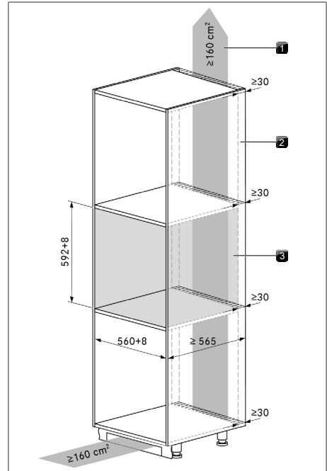
Fig. 9.1 Mobile da incasso
