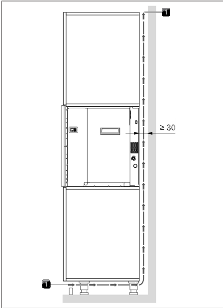
Fig. 9.17 Areazione
