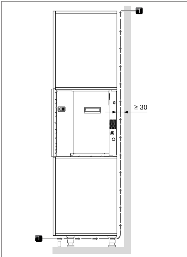
Fig. 9.16 Ventilación
