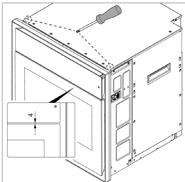
Fig. 9.14 Ajuste de la distancia entre la unidad de mando y la puerta
