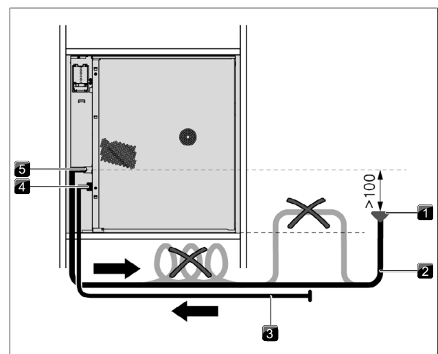
Fig. 9.11 Drenaje del agua
