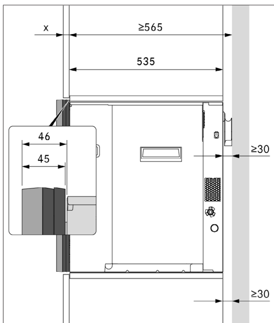
Fig. 9.5 Medidas de montaje con 2 espaciadores del marco
