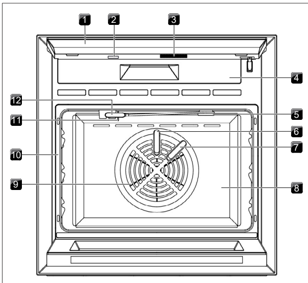
Fig. 4.1 Estructura parte 1
