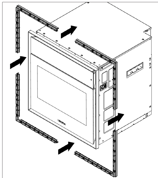
Fig. 9.6 Desmontar el espaciador del marco
