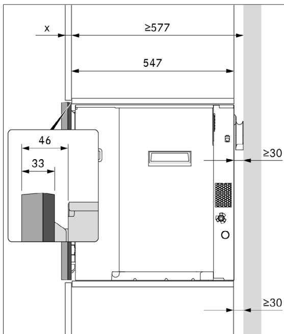
Fig. 9.4 Medidas de montaje con 1 espaciador del marco
