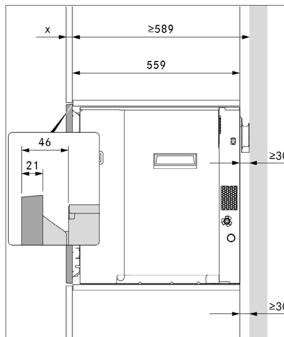
Fig. 9.3 Medidas de montaje sin espaciador del marco
