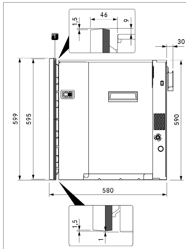
Fig. 9.2 Medidas del aparato
