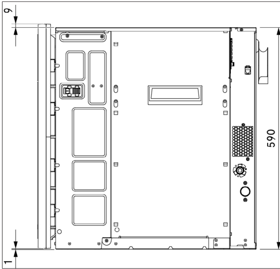
Fig. 3.3 Vista lateral XBO
