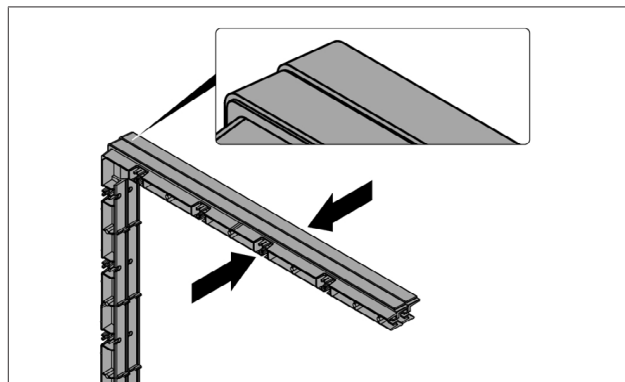
Fig. 9.7 2 espaciadores del marco
