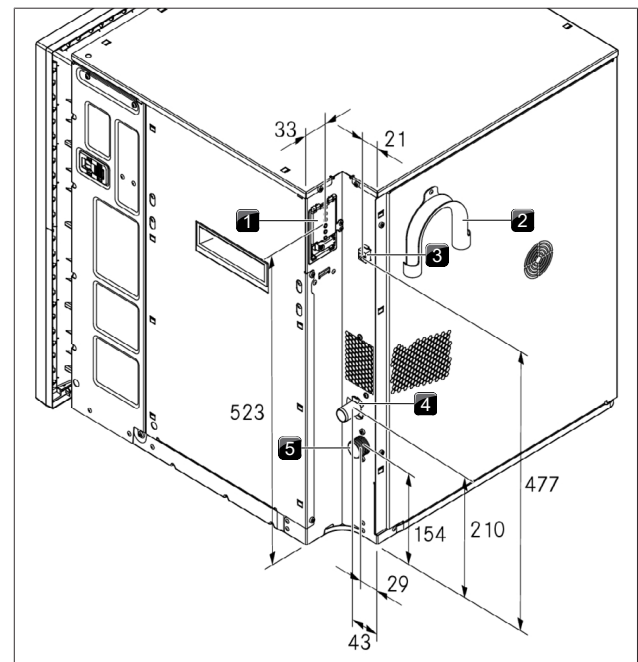
Fig. 9.10 Conexiones de aparatos
