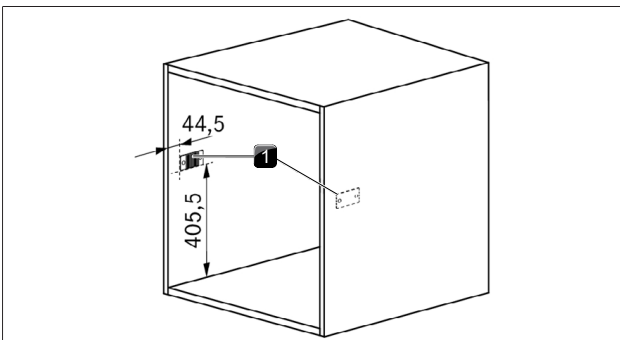
Fig. 9.9 Nicho de montaje con placas de cierre del módulo
