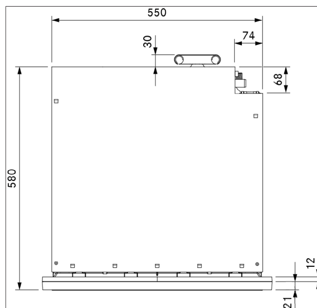
Fig. 3.2 Vista superior XBO
