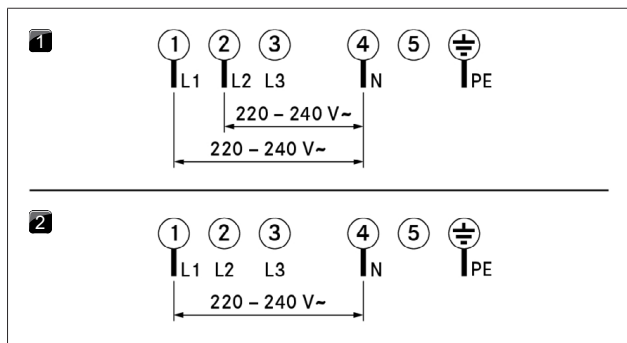
Fig. 9.13 Esquemas de conexión
