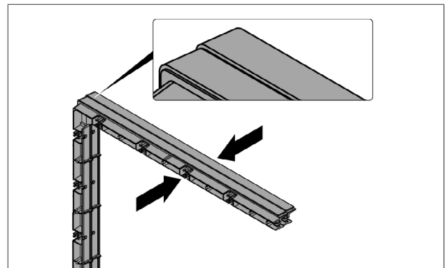
Fig. 9.7 2 frame spacers
