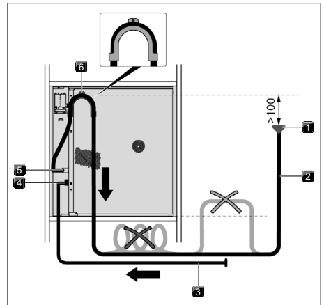
Abb. 9.12 Wasserablauf über Haltebogen
