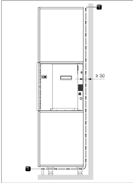
Abb. 9.17 Belüftung
