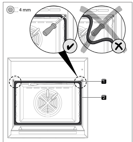
Abb. 9.16 Gerät befestigen
