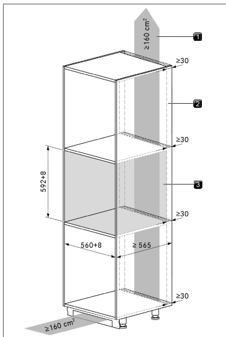
Abb. 9.1 Einbauschränk
