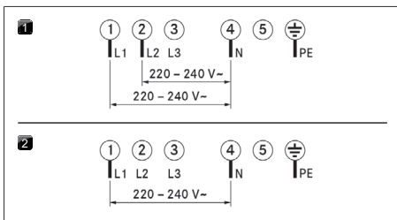
Abb. 9.14 Anschlussschemata
