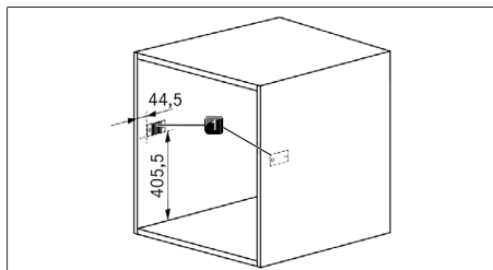
Abb. 9.9 Einbaunischie mit Korpusrastplatten
