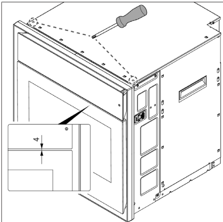
Abb. 9.15 Einstellung Abstand Bedieneinheit und Tür
