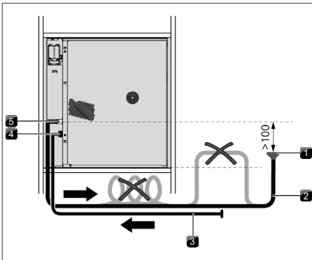
Abb. 9.11 Wasserablauf
