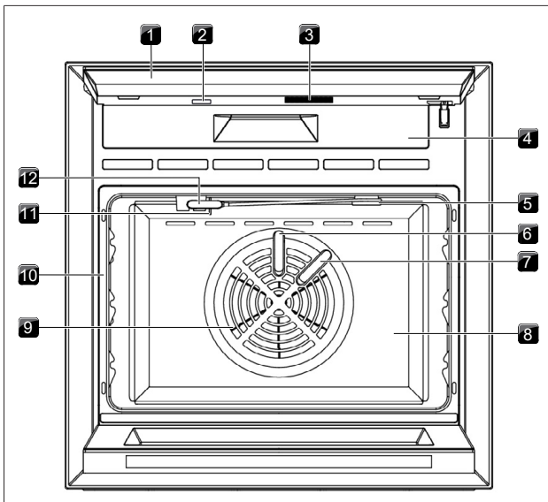
Abb. 4.1 Aufbau Teil 1
