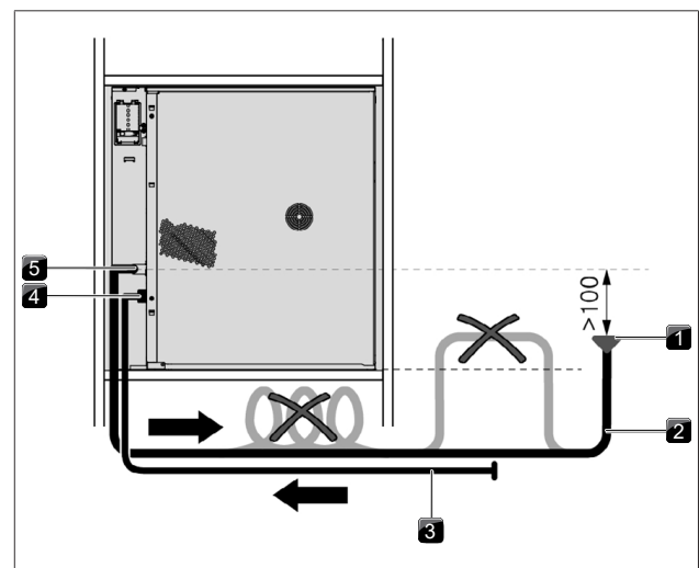
Abb. 9.11 Wasserablauf
