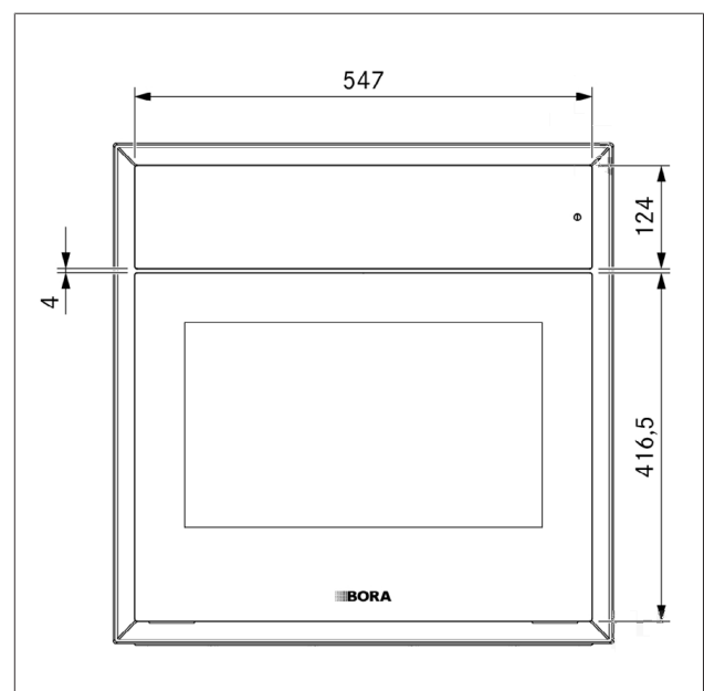
Abb. 3.4 Vorderansicht Glas XBO
