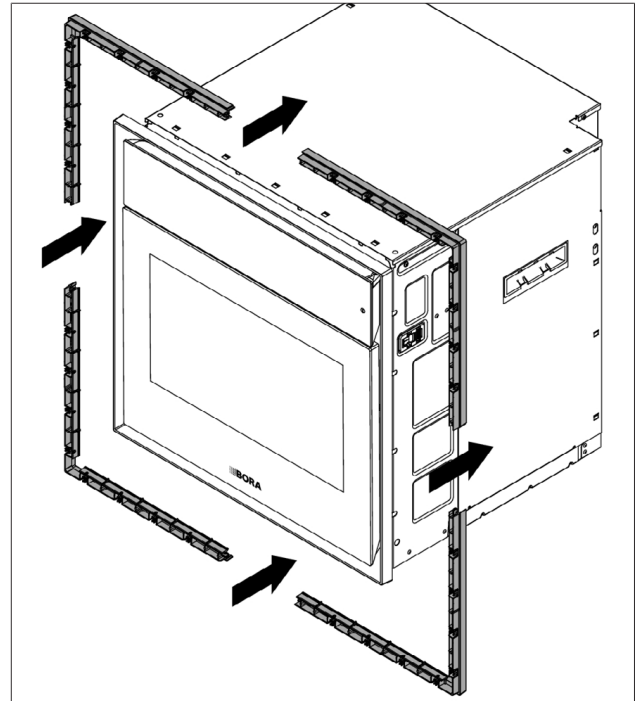
Abb. 9.6 Rahmen Spacer demontieren
