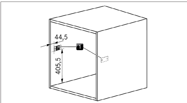
Abb. 9.9 Einbaunische mit Korpusrastplatten
