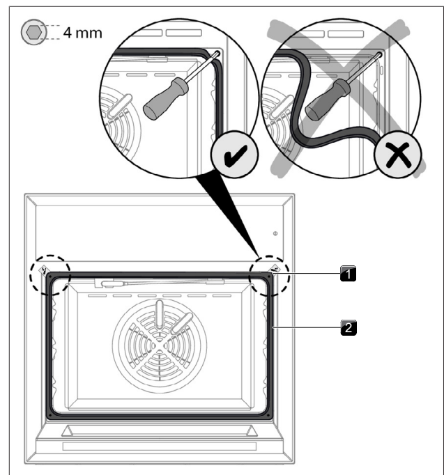
Abb. 9.15 Gerät befestigen
