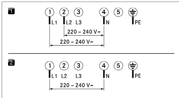
Abb. 9.13 Anschluss schemata
