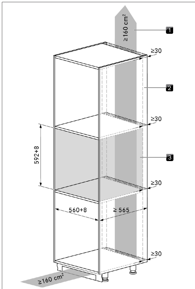
Abb. 9.1 Einbauschrank
