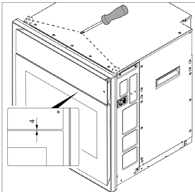
Abb. 9.14 Einstellung Abstand Bedieneinheit und Tür
