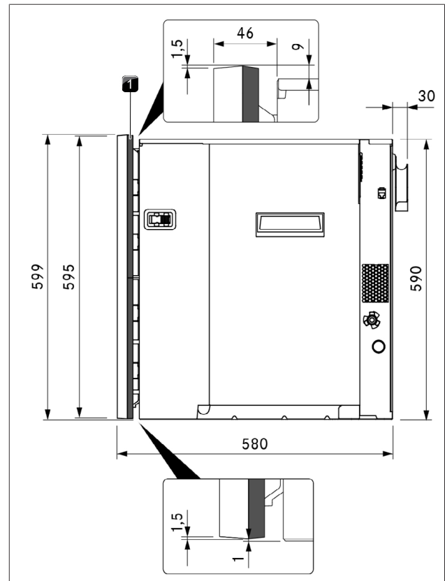
Abb. 9.2 Gerätemaße
