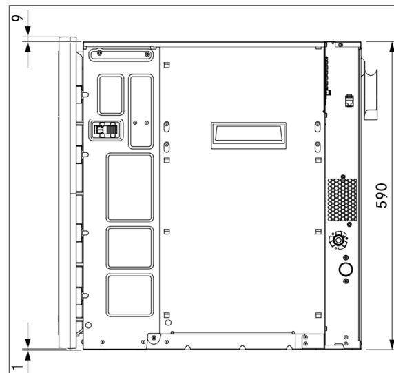
Abb. 3.3 Seitenansicht XBO
