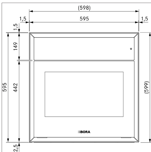
Abb. 3.1 Vorderansicht XBO
