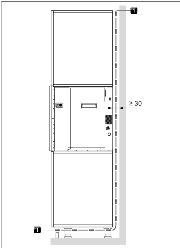
Abb. 9.16 Belüftung
