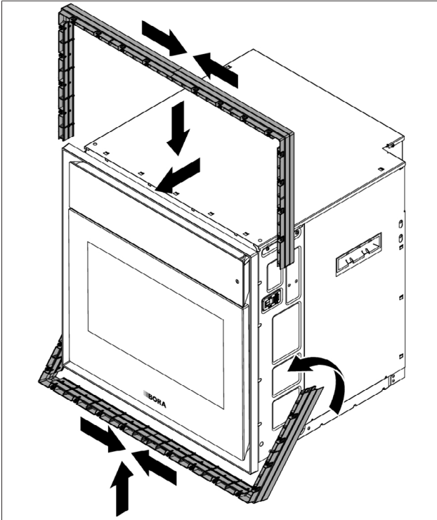
Abb. 9.8 2 Rahmen Spacer montieren
