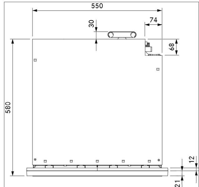
Abb. 3.2 Draufsicht XBO
