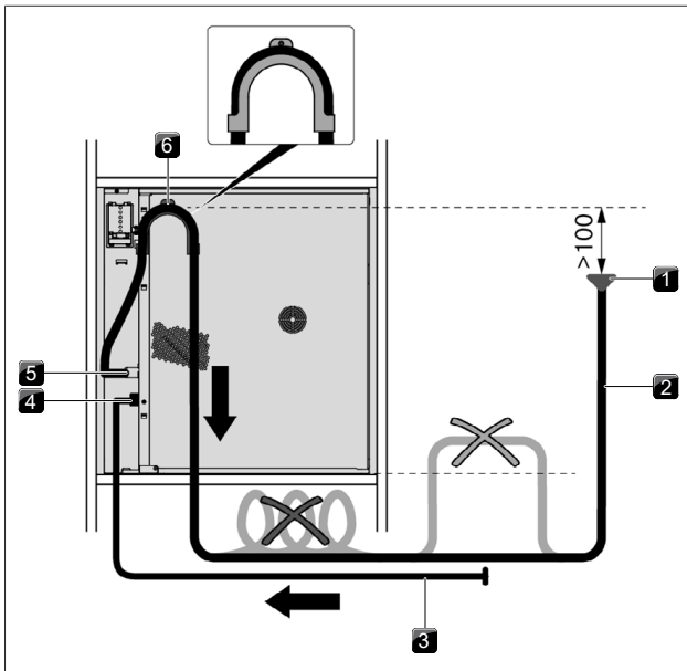
Abb. 9.12 Wasserablauf über Haltebogen
