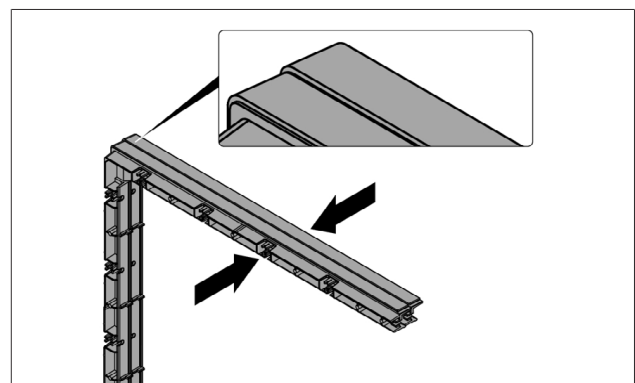
Abb. 9.7 2 Rahmen Spacer-Elemente
