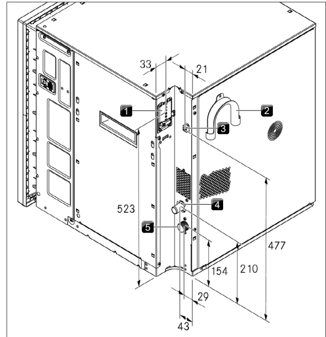
Abb. 9.10 Geräteanschlüsse
