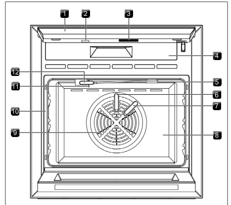
Fig. 4.1 Opbygning del 1
