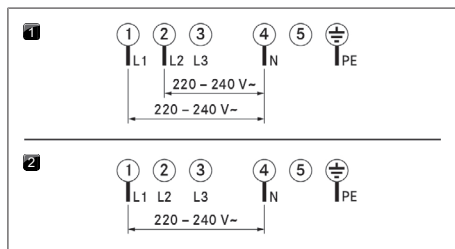
Fig. 9.14 Tilslutningsskema
