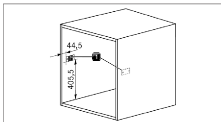
Fig. 9.9 Installationsniche med kabinetlåseplade
