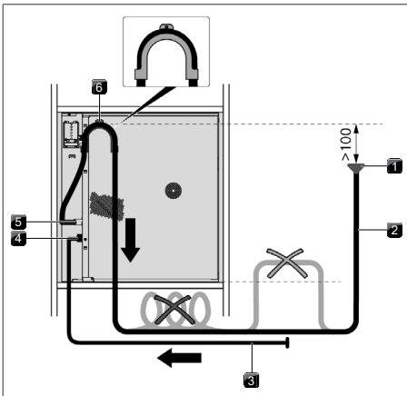
Fig. 9.12 Vandafløb over holdebøjlen
