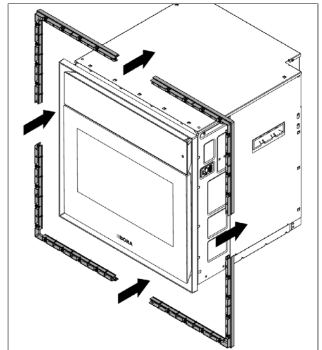
Fig. 9.6 Afmontering af afstandsramme
