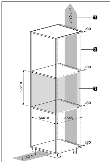
Fig. 9.1 Indbygningskabinet
