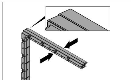
Fig. 9.7 2 afstandsrammeelementer
