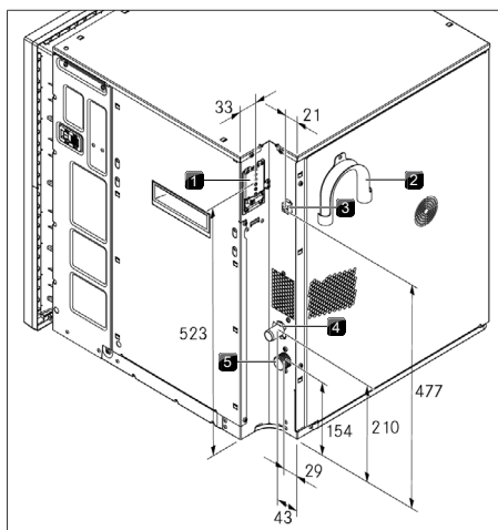
Fig. 9.10 Tilslutnings af apparater
