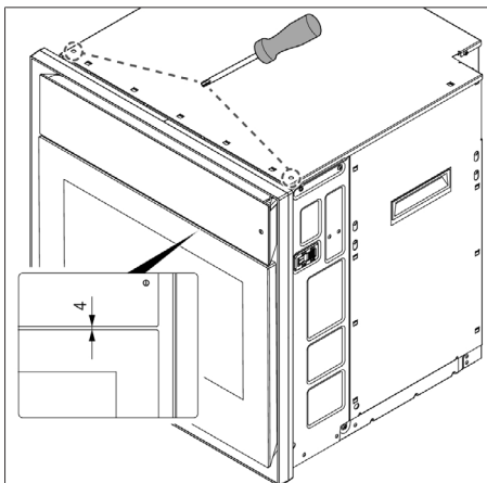
Fig. 9.15 Indstilling af afstanden mellem betjeningsenheden og døren
