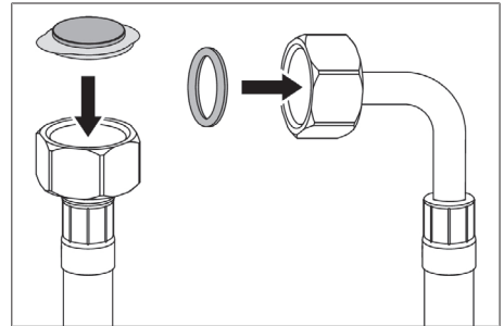
Fig. 9.13 Vandtilløbslange med snavssi og pakning
