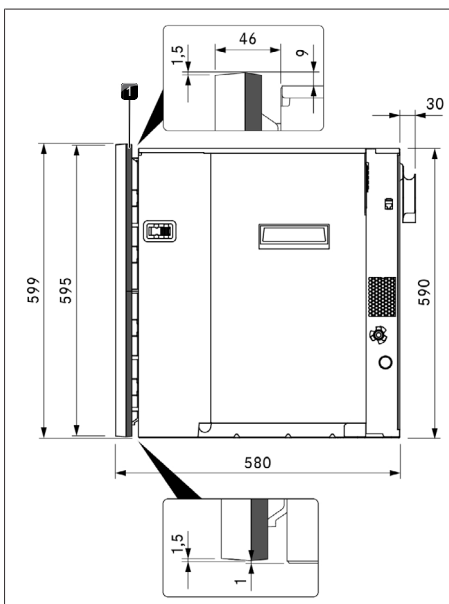
Fig. 9.2 Apparatmål
