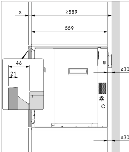
Fig. 9.3 Indbygningsmål uden afstandsramme
